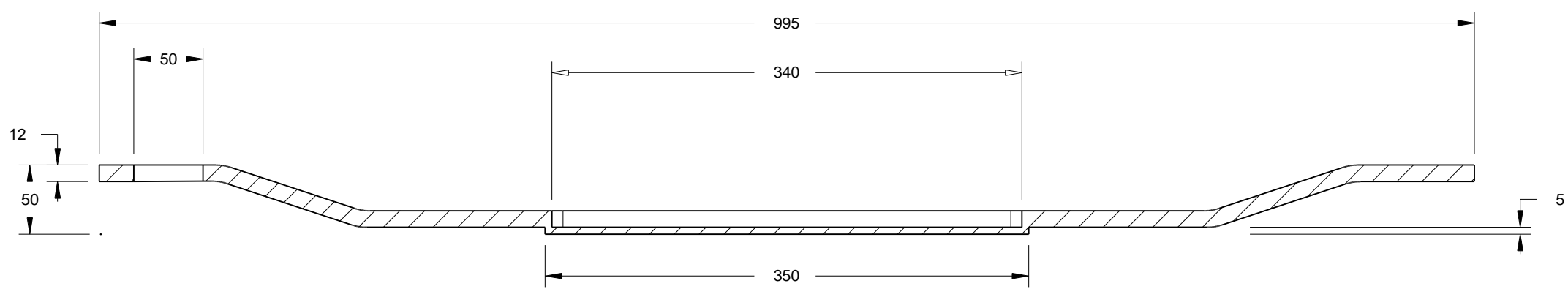
Section A-A
